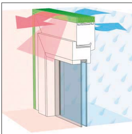
obr. 1: Funkčný princíp
